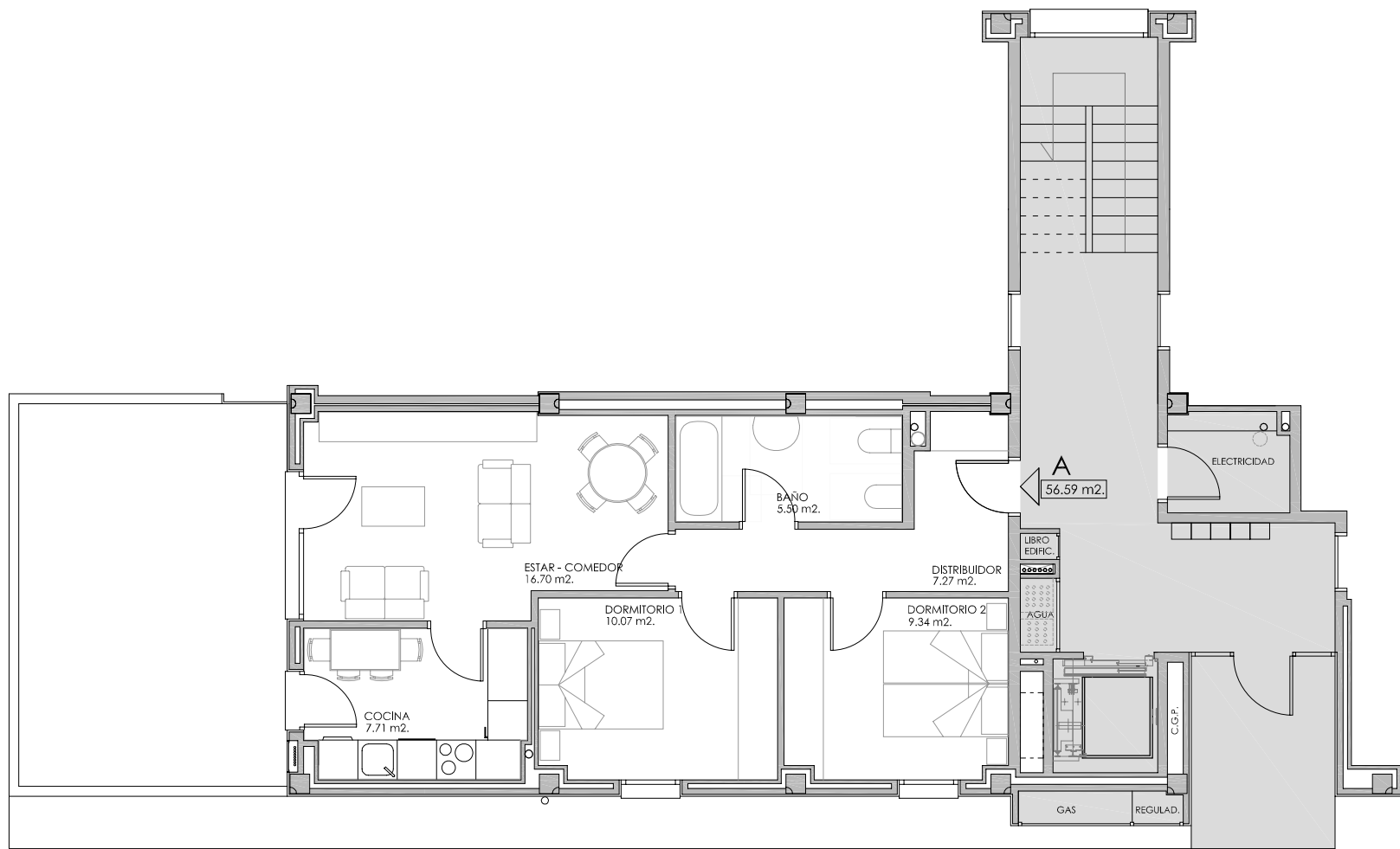
PLANTA ESCALA 1:100
